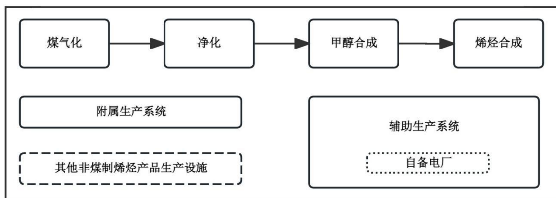
图2 核算边界示意图
