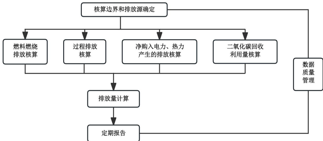
图1 工作程序
