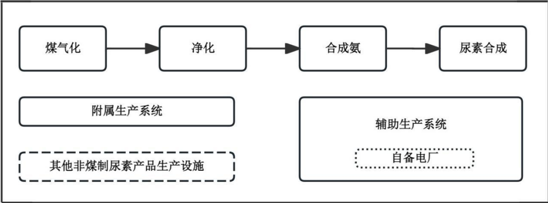
图2 核算边界示意图
